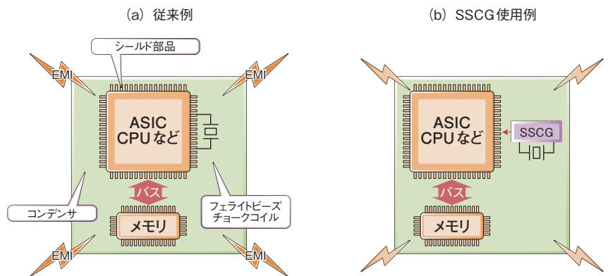
図1 従来のEMI対策とSSCG使用例
