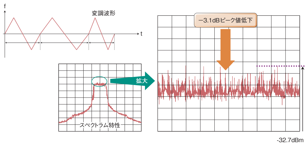
図7 富士通の複合変調技術を用いたスペクトラム波形例
