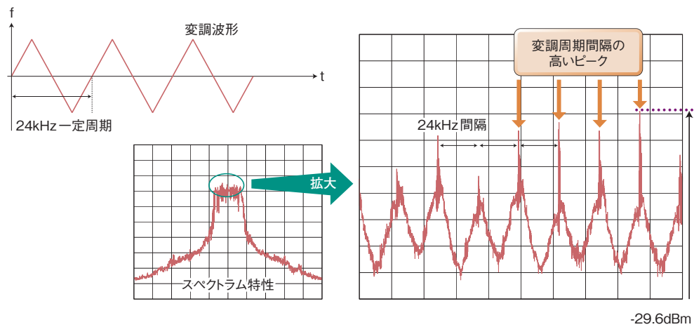
図6 単一周期で動作させた場合のスペクトラム波形例
